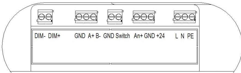
Рисунок 4. Клеммники подключения
