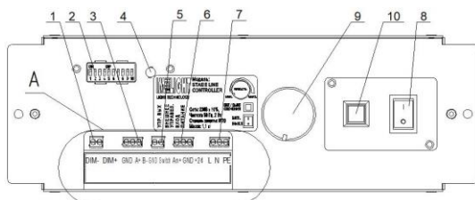
Исполнение STAGE LINE CONTROLLER
