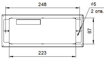
Встраиваемое исполнение STAGE LINE CONTROLLER
