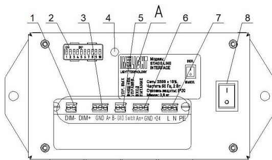
Исполнение STAGE LINE INTERFACE
