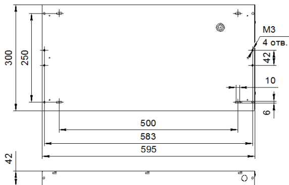
Рисунок 1. Габаритные размеры светильника
