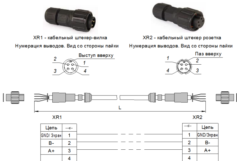
Рисунок 6. Схема разделки кабеля и распайки разъёмов
