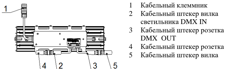
Рисунок 2. Органы управления
