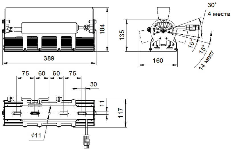
Рисунок 1. Габаритные размеры светильника
