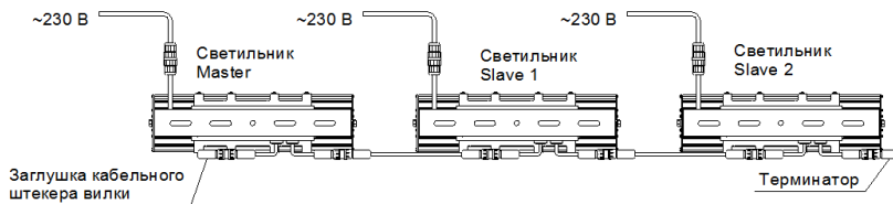
Рисунок 5. Пример подключения 3 светильников в режиме MASTER - SLAVE.
