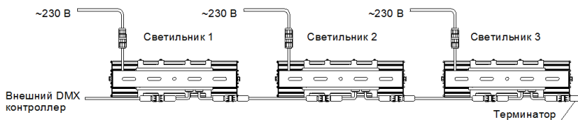
Рисунок 4. Пример подключения 3 светильников в линию DMX-512
