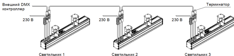
Рисунок 4. Пример подключения 3 светильников в линию DMX-512
