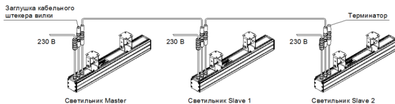
Рисунок 5. Пример подключения 3 светильников в режиме MASTER - SLAVE.
