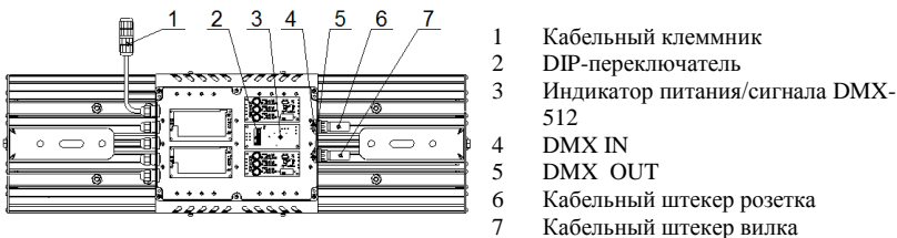
Рисунок 2 Органы управления
