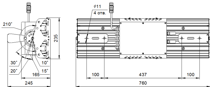
Рисунок 1 Габаритные размеры светильника
