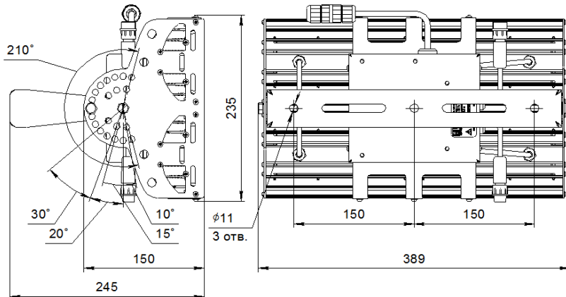
Рисунок 1. Габаритные размеры светильника
