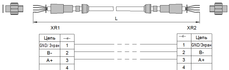
Рисунок 5. Схема разделки кабеля и распайки разъемов DMX/RDM IN/OUT
